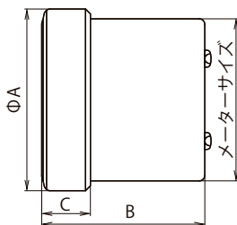
【メーター側面】
