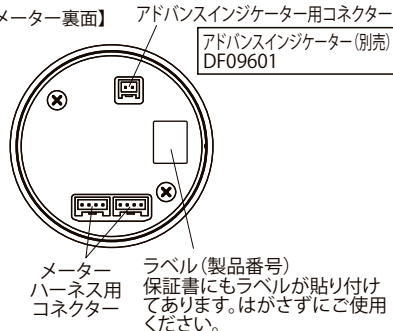
【メーター裏面】
