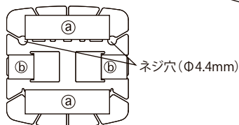
【図4】 取付金(裏面)
